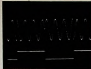
Afb. 15. Fasemodulatie (PSK = phase-shift keyed) Realisatie: 1-sweep-blok symmetrisch om nul-lijn. 2-VCO. 3-beide signalen in analoge vermenigvuldiger.
